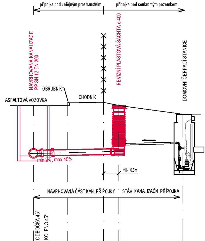
PODÉLNÝ PROFIL
