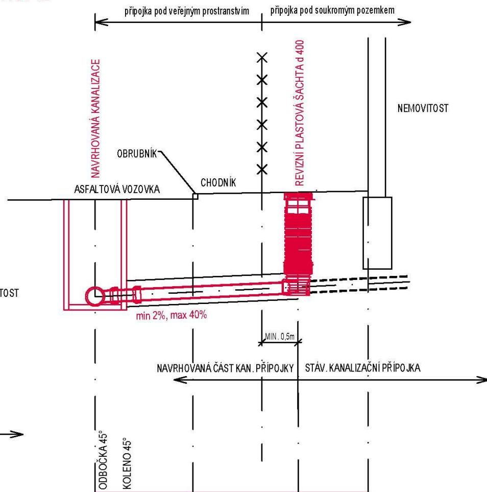
PODÉLNÝ PROFIL
