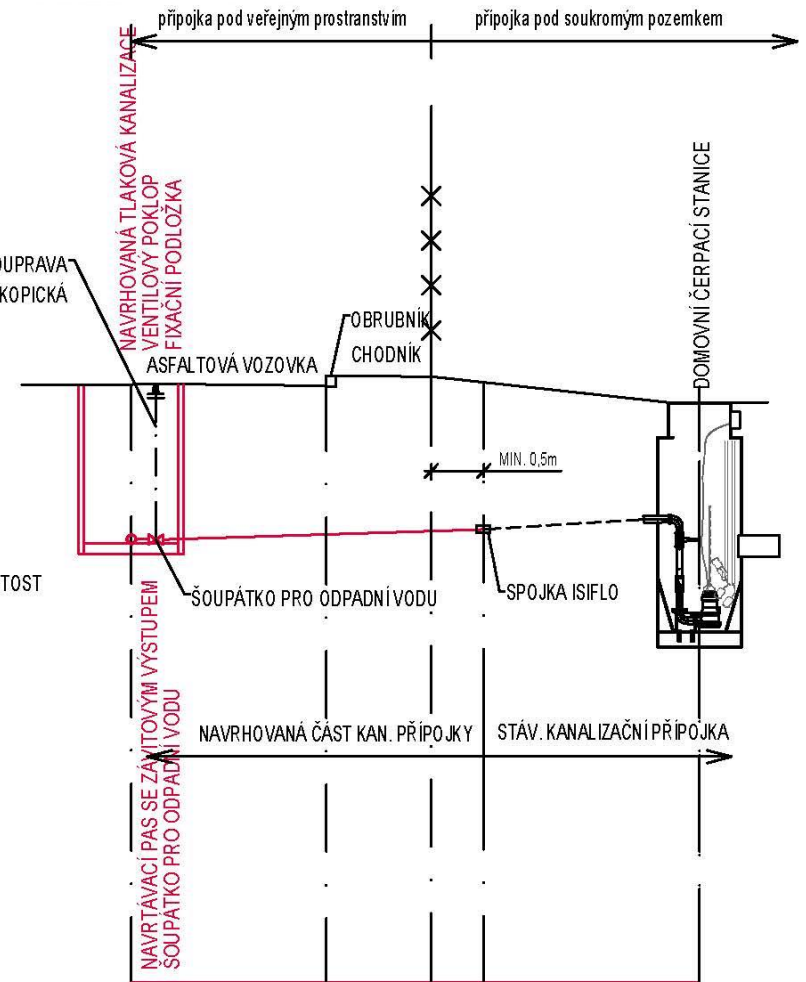
PODÉLNÝ PROFIL
